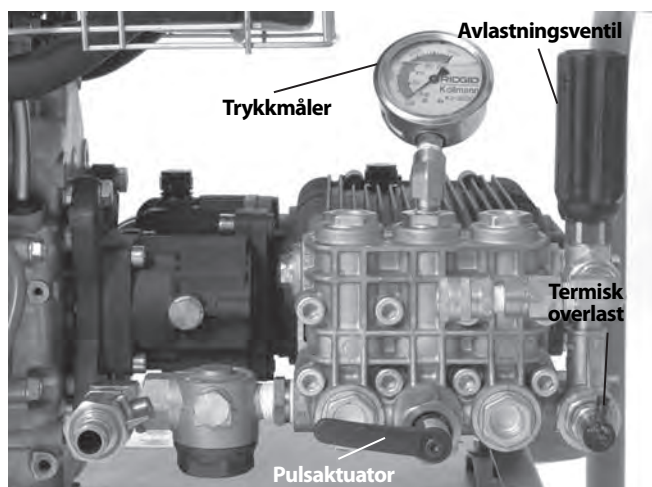
Figur 13 – Kontroller
