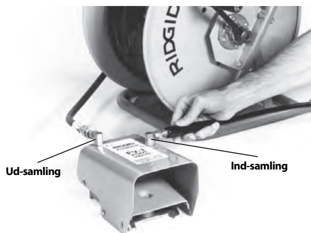
Figur 11 – Fodventiltilslutning
