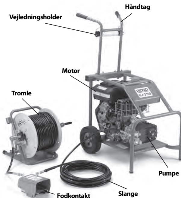
Figur 2 – KJ-3100-højtryksrensemaskine
