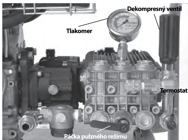
Obrázok č. 13 - Ovládacie prvky
