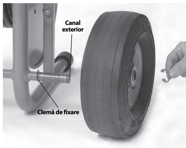
Figura 4 – Asamblarea KJ-2200
