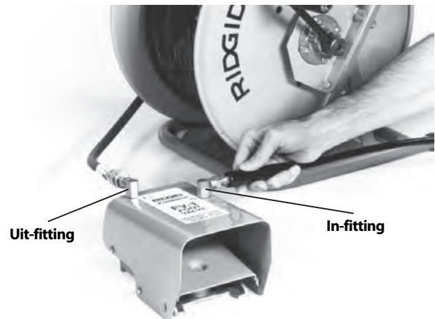
Figuur 11 – Voetklepaansluiting
