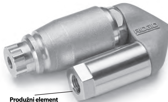
Slika 12 – Mlaznica RR3000 s produžnim elementom
