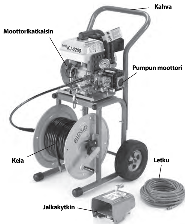
Kuva 1 – KJ-2200 Painehuuhtelulaite
