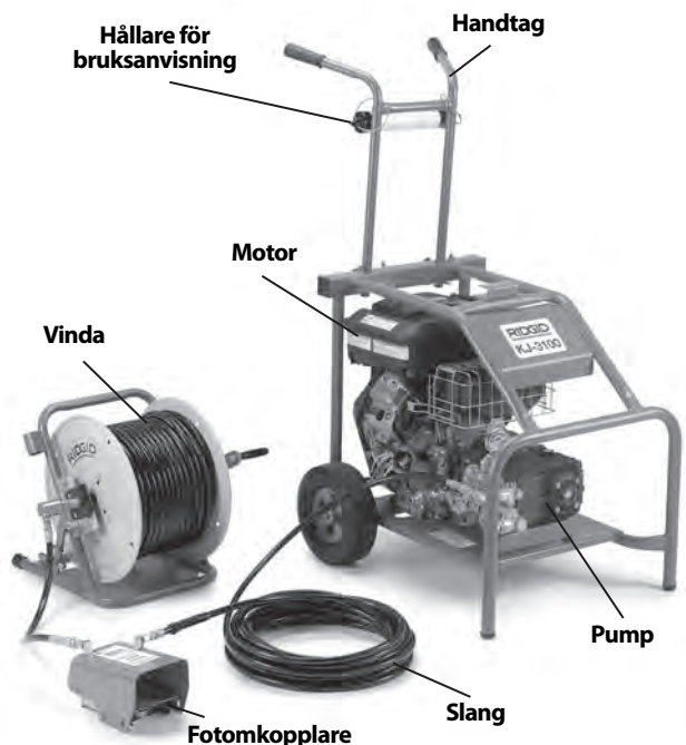
Figur 2 – KJ-3100 Högtrycksrensare (vatten)
