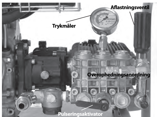
Figur 13 – Kontroltaster
