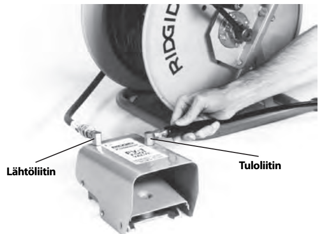
Kuva 11 – Jalkaventtiiliin liittäminen
