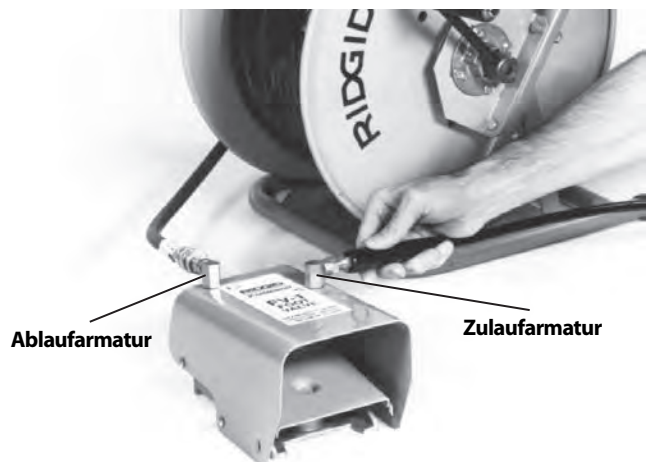
Abbildung 11 – Fußventilanschluss
