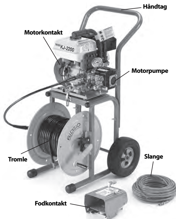
Figur 1 – KJ-2200-højtryksrensemaskine
