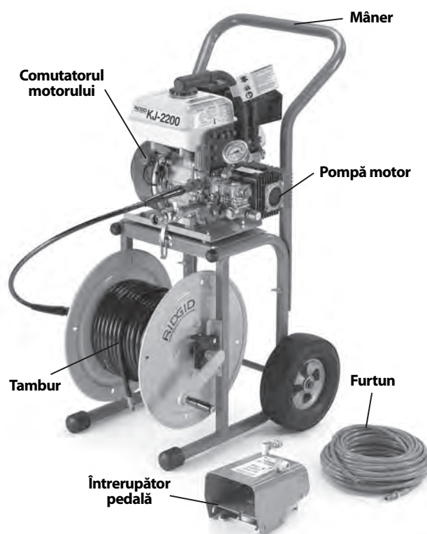
Figura 1 – Mașina cu jet de apă KJ-2200
