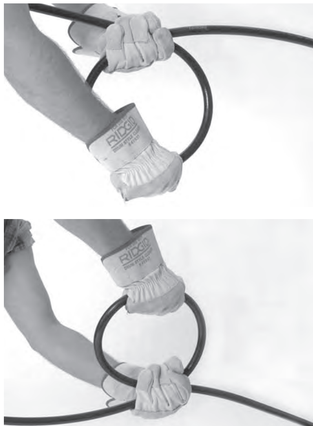
Рис. 15 – Вращение шланга
