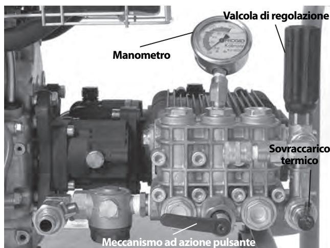
Figura 13 – Comandi
