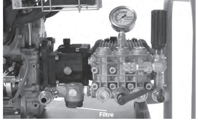
Şekil 7 – Giriş Filtresi/Filtre Pulı
