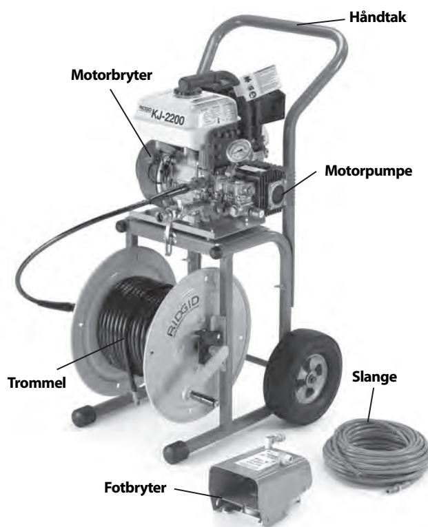
Figur 1 – KJ-2200 høytrykksspyler
