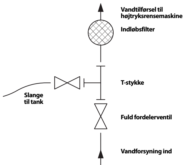
Figur 9 – Vandtilførselstilslutninger ved brug af tank
