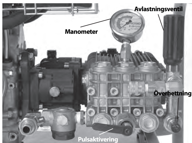
Figur 13 – Reglage
