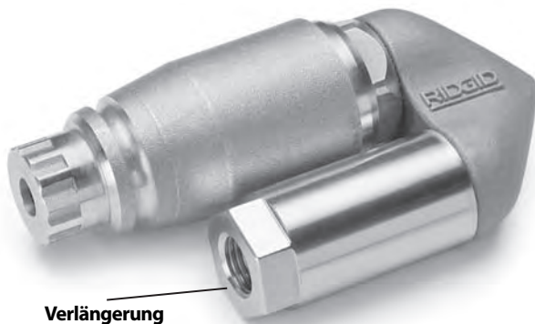
Abbildung 12 – RR3000 Düse mit Verlängerung
