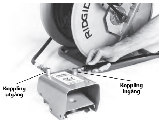
Figur 11 – Anslutning av fotventil
