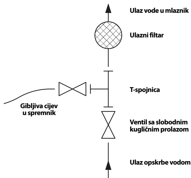
Slika 9 – Priključci na dovod vode kod uporabe spremnika
