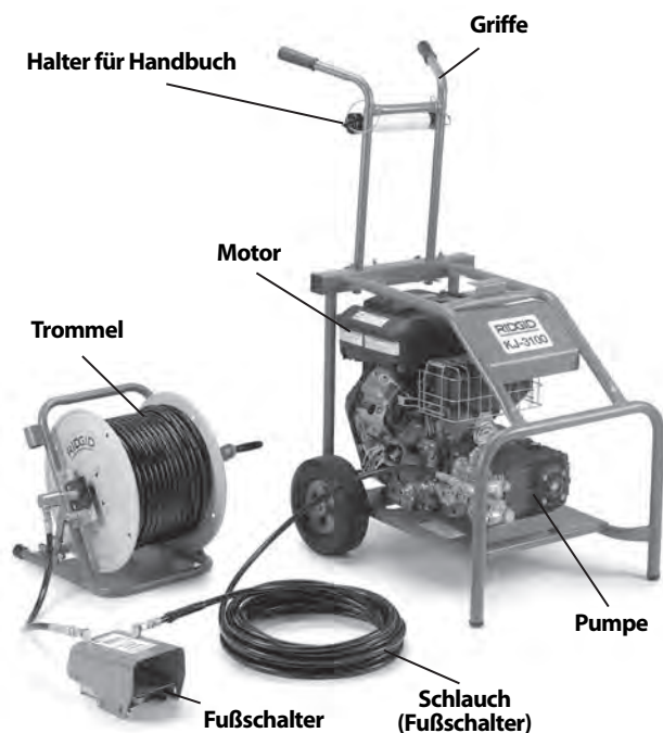
Abbildung 2 – KJ-3100 Hochdruck-Rohrreiniger
