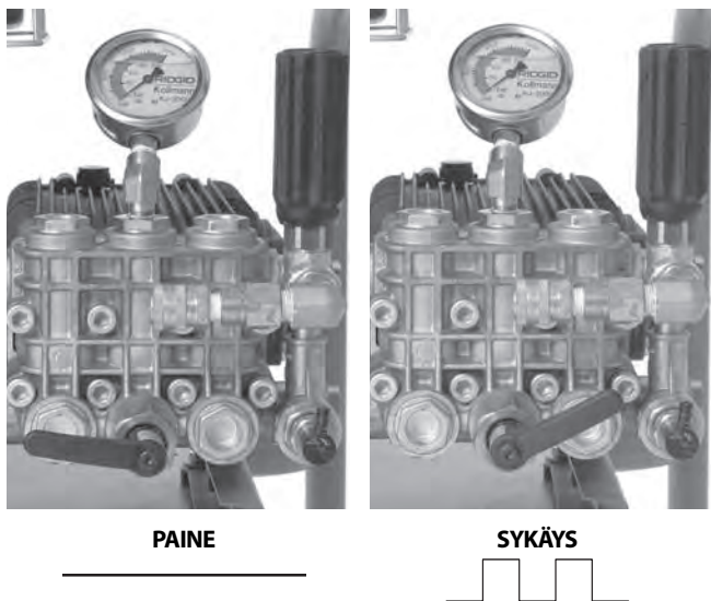
Kuva 16 – Sykäskäyttölaitteen vivun asento
