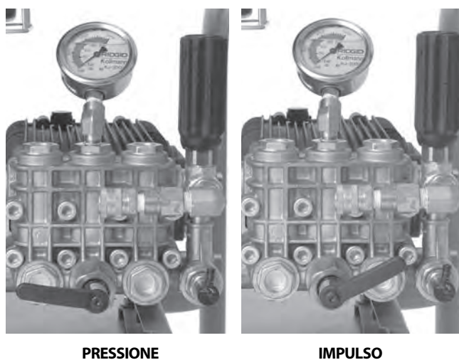
Figura 16 – Posizione della leva del meccanismo ad azione pulsante
