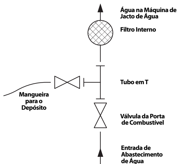
Figura 9 - Ligações de Abastecimento de Água quando Utilizar um Depósito
