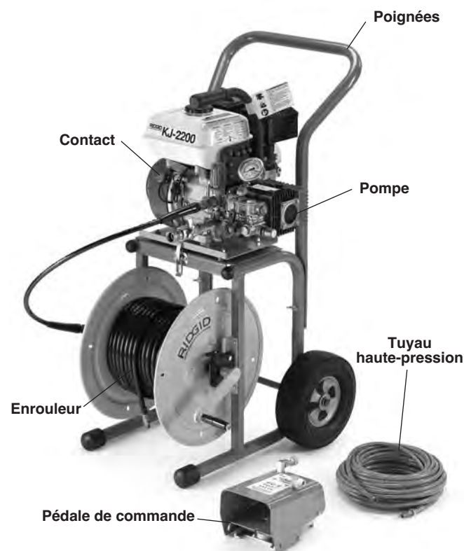
Figure 1 – Dégorgeoir haute-pressure KJ-2200
