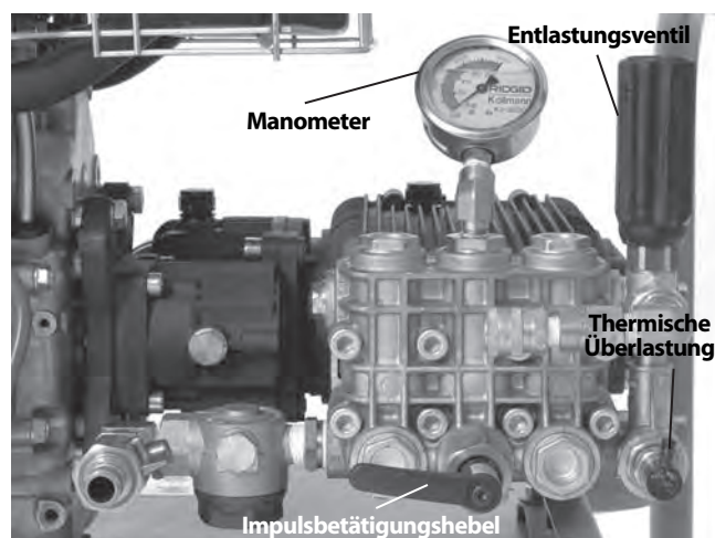
Abbildung 13 – Bedienelemente
