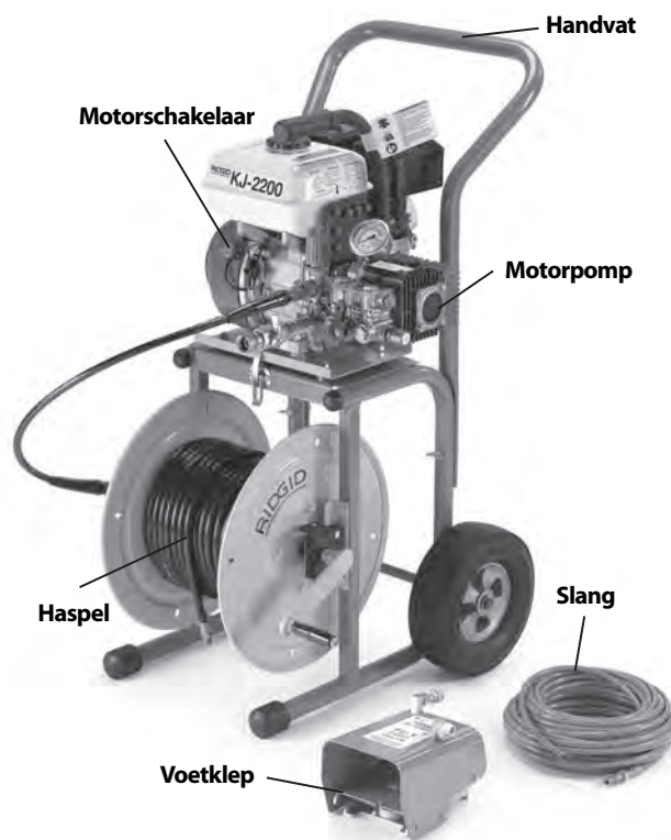
Figuur 1 – KJ-2200 Hogedrukrioolreiniger
