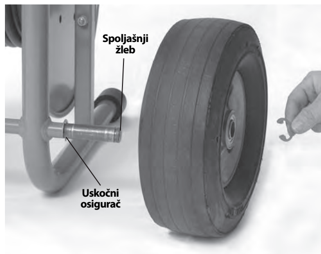
Slika 4 – Sklop KJ-2200
