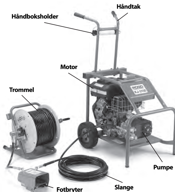
Figur 2 – KJ-3100 høytrykksspyler
