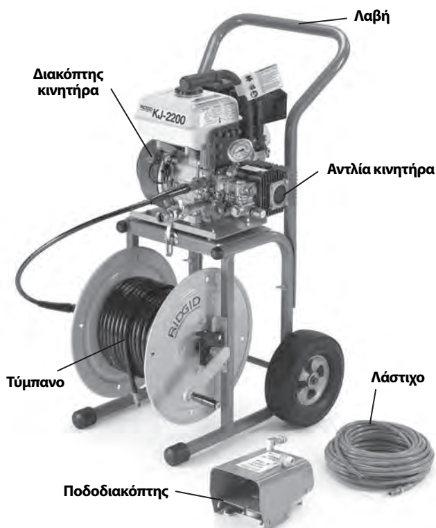
Εικόνα 1 – Πιεστικό νερού KJ-2200
