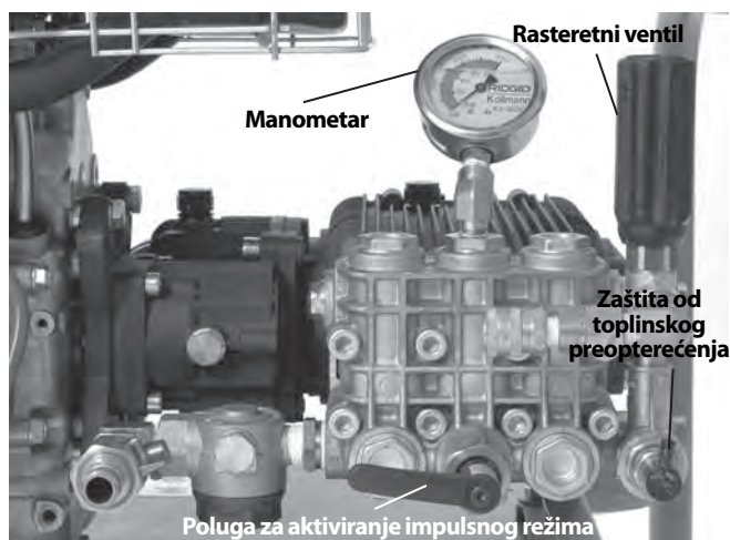
Slika 13 – Kontrole
