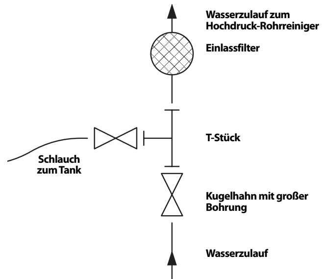
Abbildung 9 – Wasserzufuhranschlüsse bei Benutzung eines Tanks
